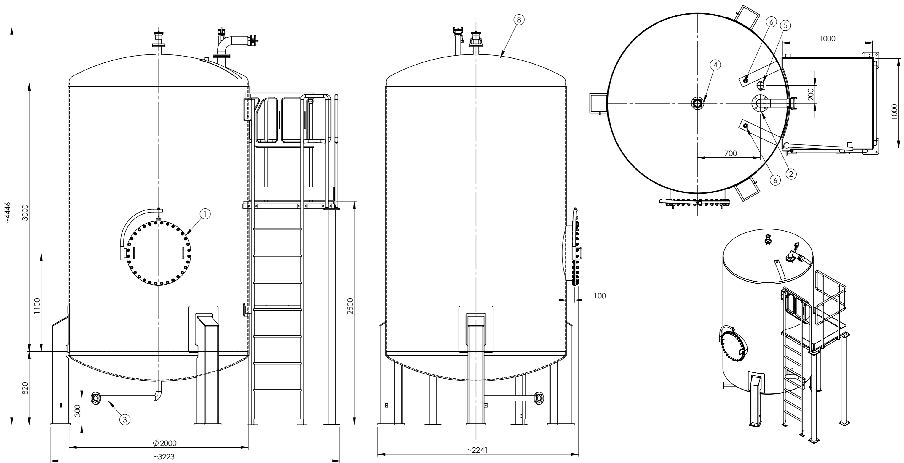
Zbiornik V-10m 3 Nziemny pionowy, jednokomorowy, dwupłaszczowy do oleju opałowego Rysunek informacyjny/ofertowy. Nr rys.: ZN1-2,0/10-OF37/17
